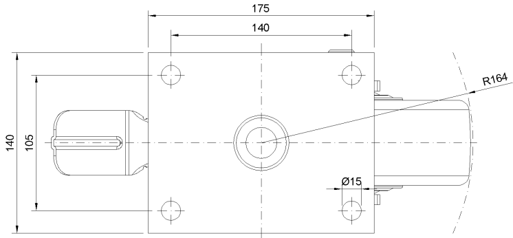
Bản vẽ chỉ mang tính chất tham khảo có thể khác với sản phẩm thực tế.
