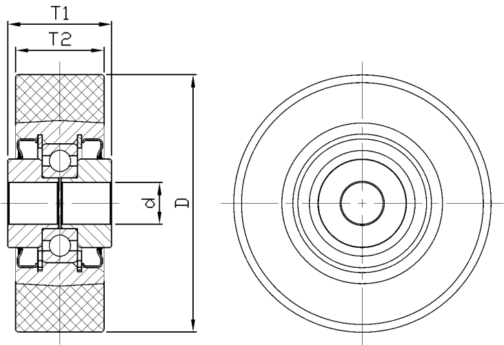
Bản vẽ 2D phác thảo kích thước bánh xe đơn
