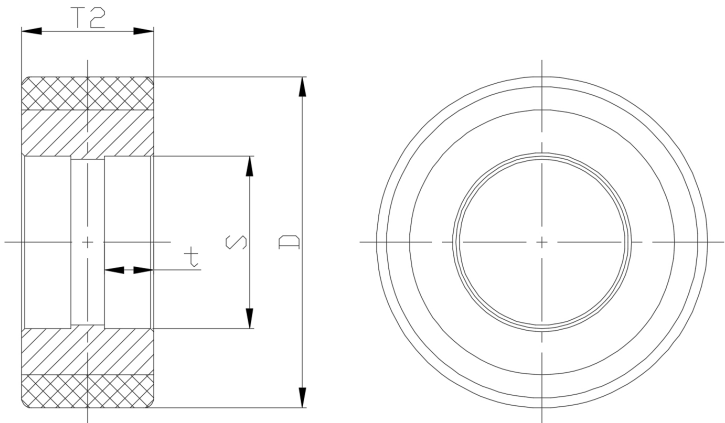
Bản vẽ 2D phác thảo kích thước bánh xe đơn
