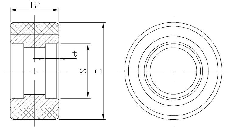
Bản vẽ 2D phác thảo kích thước bánh xe đơn
