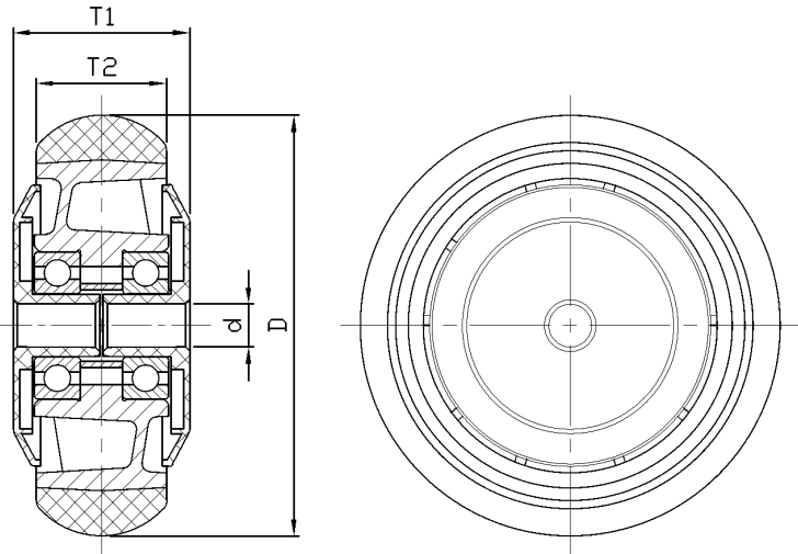
Bản vẽ 2D phác thảo kích thước bánh xe đơn
