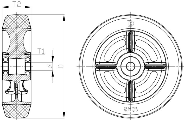
Bản vẽ 2D phác thảo kích thước bánh xe đơn
