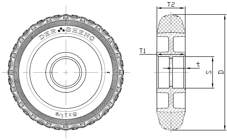
Bản vẽ 2D phác thảo kích thước bánh xe đơn
